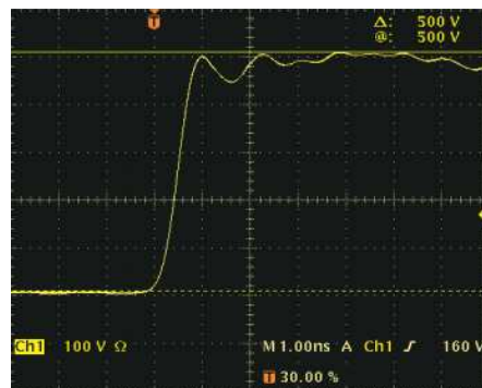
500V/div. 1ns/div
