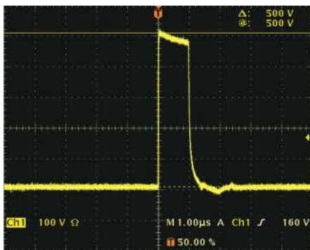
500V/div. 1µs/div
